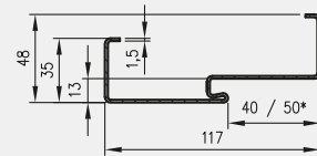
Przekrój ościeżnicy metalowej p.poż. do skrzydeł OLIMP
