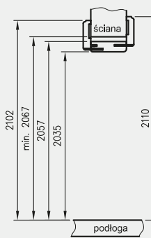
Przekrój pionowy tunelu regulowanego z ką. K63 lub N63
