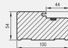
Przekrój poziomy ościeżnicy w murze
