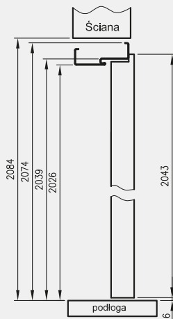
Przekrój pionowy drzwi p.poż.
