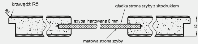
Przekrój poziomy drzwi VETRO B5, B8-B11
