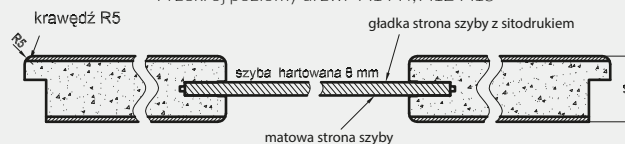
Przekrój poziomy drzwi A1-A4, A12-A15
