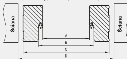
przekrój poziomy ościeżnicy w murze
