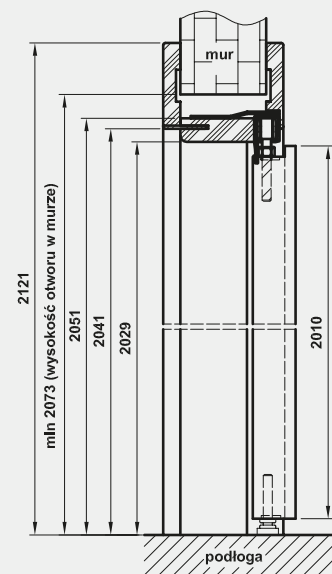
Przekrój pionowy
