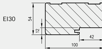
Przekrój ościeżnicy drewnianej p.poż do skrzydeł OLIMP
