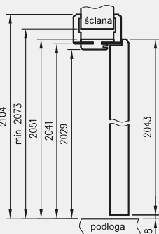
Przekrój OR/ORC Natura z ką. N63
