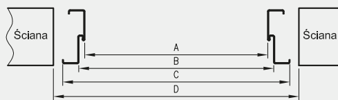
Przekrój poziomy ościeżnicy w murze
