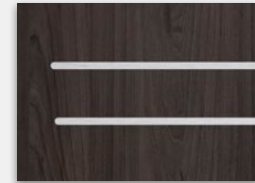
wstawki aluminiowe o przekroju 8x2 mm umiejscowione w jednej płaszczyźnie z powierzchnią drzwi
