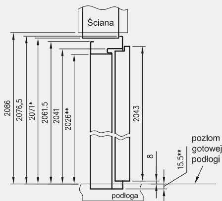
Przekrój pionowy
