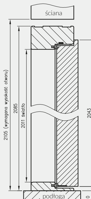
przekrój pionowy drzwi Forca
