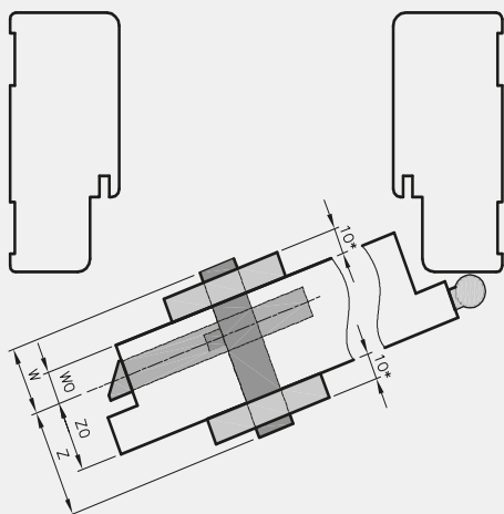
Rys. Dobór wymiaru wkładki bębnekowej
