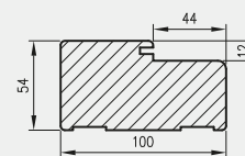
przekrój poziomy ościeżnicy w murze
