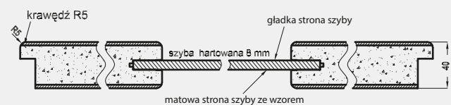
Przekrój poziomy drzwi VETRO B5, B8-B11
