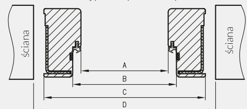
Przekrój poziomy ościeżnicy w murze
