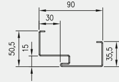
Profil ościeżnicy metalowej
