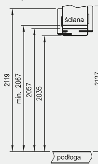
Przekrój pionowy tunelu regulowanego z ką. T80
