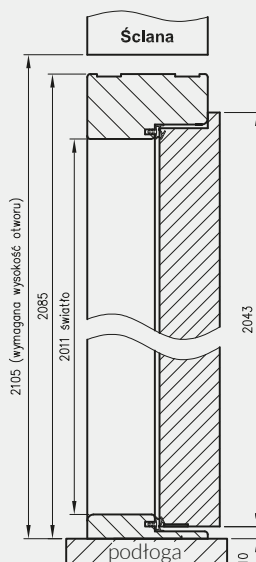
przekrój pionowy drzwi Athos
