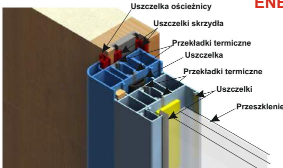
SKRZYDŁO KMT PLUS 75 passive PROFIL OŚCIEŻNICY ENERGY 90 + PROFIL NAŚWIETLA
