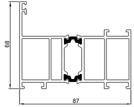
Profil proggu ENERGY 90
