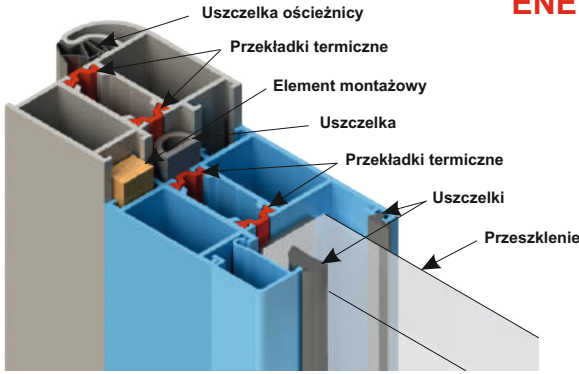
PROFIL OŚCIEŻNICY ENERGY 60 PROFIL NAŚWIETLA ENERGY 60
