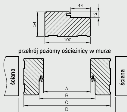
przekrój ościeżnicy drewnianej p.poż. do skrzydeł Athos
