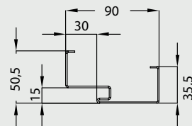
Profil ościeznicy metalowej
