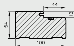
Przekrój poziomy ościeżnicy w murze
