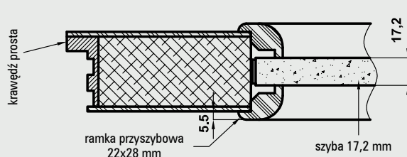
konstrukcja skrzydeł przeciwpożarowych Olimp EI30
