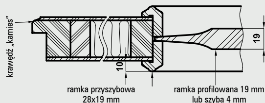
konstrukcja skrzydeł przylgowych Cell kolekcja Classic
