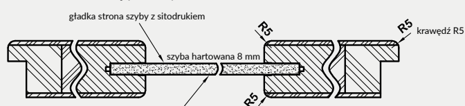
Przekrój poziomy drzwi VETRO B5, B10-B11
