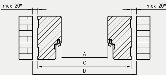
Przekrój poziomy OD ATHOS
