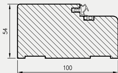
Profil OD ATHOS
