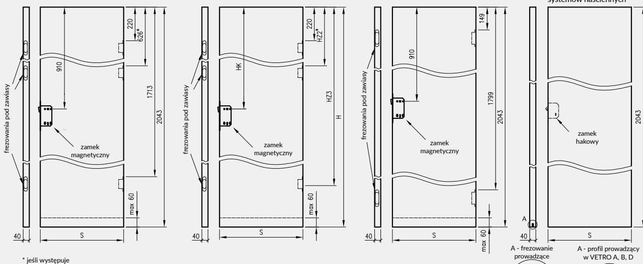
Skrzydła bezprzylgowe rozwiernie Standard 10, Modern, Plus
