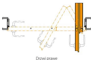
SPOSÓB OTWIERANIA DRZWI (rzut z góry)
