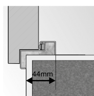
ościeżnica kątowa mała
