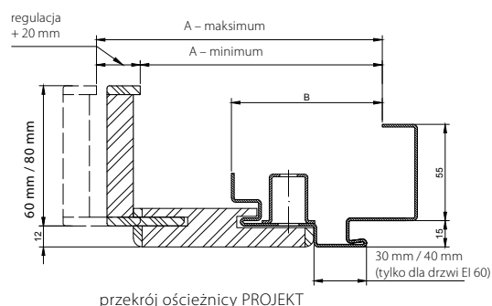
przekrój ościeżnicy PROJEKT
