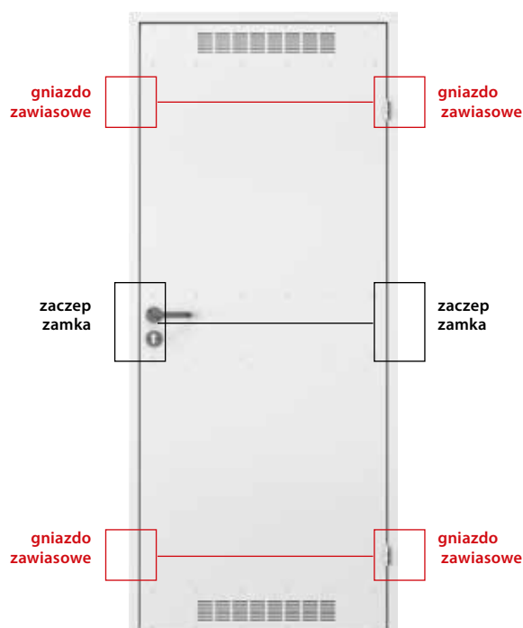
przód skrzydła
