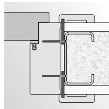
montaż na wkręty w ścianie z płyty kartonowo-gipsowej
