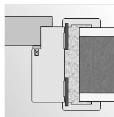
montaż na piankę w ścianie murowanej
