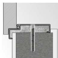
ościeżnica kątowa duża montaż na dyble
